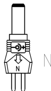
Hohlstecker/ hollowplug \varnothing 1,5 \times \varnothing 5,5 \times 12 \text{ mm}
