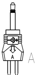
Klinkenstecker/ jackplug \varnothing 2,5 \times 13 \pm 0,5 \text{ mm}
