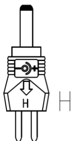
Hohlstecker/ hollowplug \varnothing 1,35 \times \varnothing 3,5 \times 10 \text{ mm}
