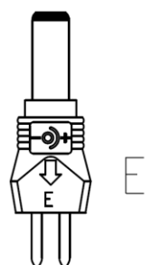
Hohlstecker/ hollowplug \varnothing 2,1 \times \varnothing 5,5 \times 12 \text{ mm}
